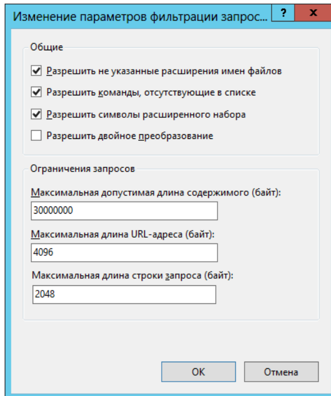
Рис. 161 – Параметры фильтрации запросов
