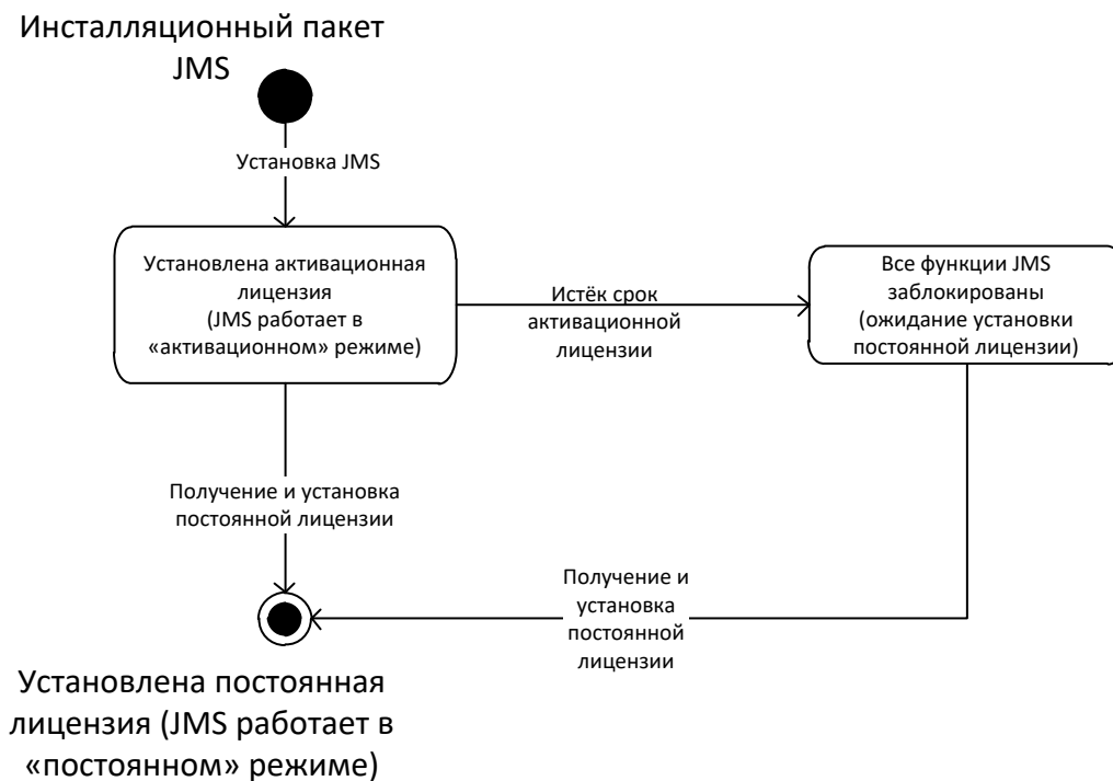
Рис. 201 – Диаграмма переходов для процедуры активации JMS
