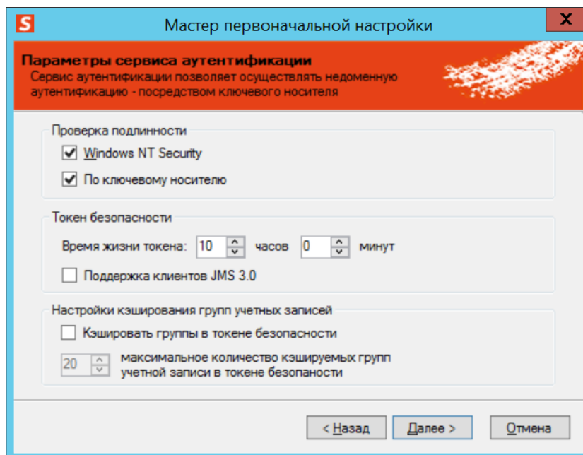
Рис. 94 – Настройка службы аутентификации JMS
