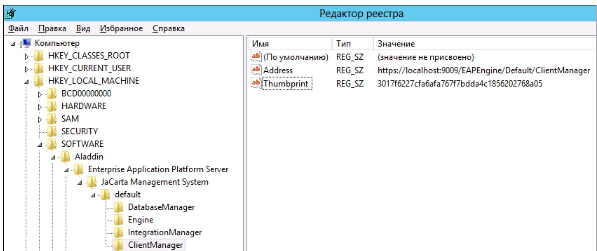
Рис. 139 – Настройки для клиентского агента из состава JMS Client
