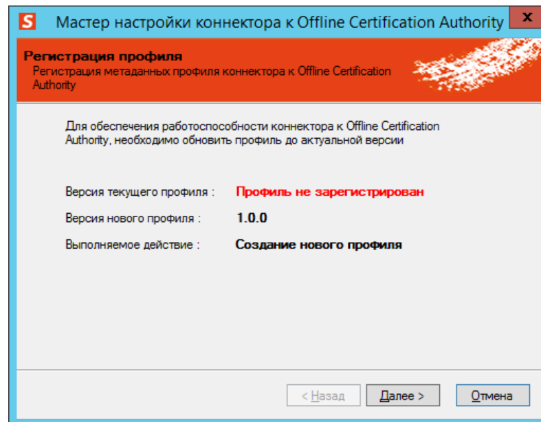
Рис. 236 – Окно запроса на обновление профиля коннектора
