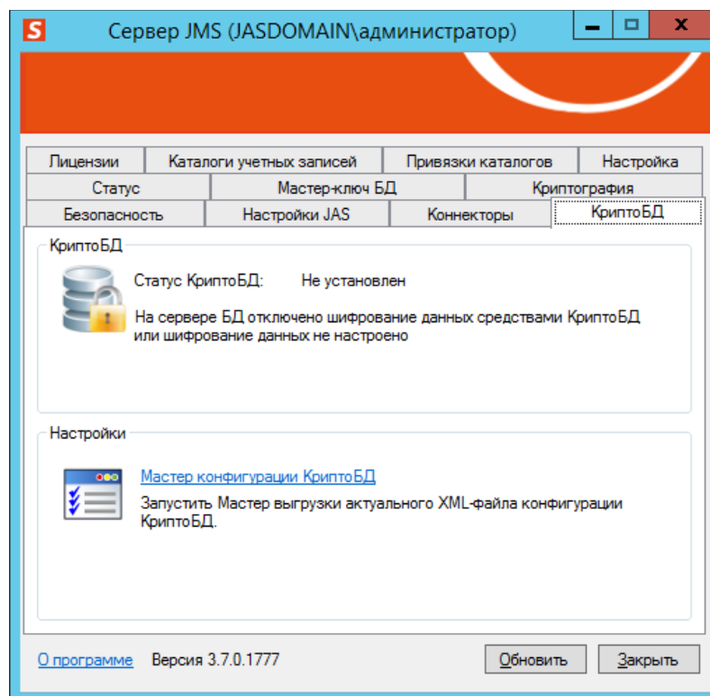
Рис. 243 – Добавление вкладки КриптоБД в серверном агенте JMS
