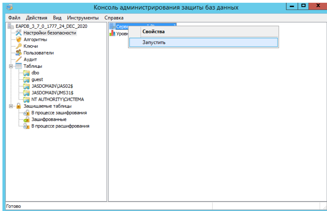
Рис. 264 – Запуск сервера ключей СКЗИ «Крипто БД»
