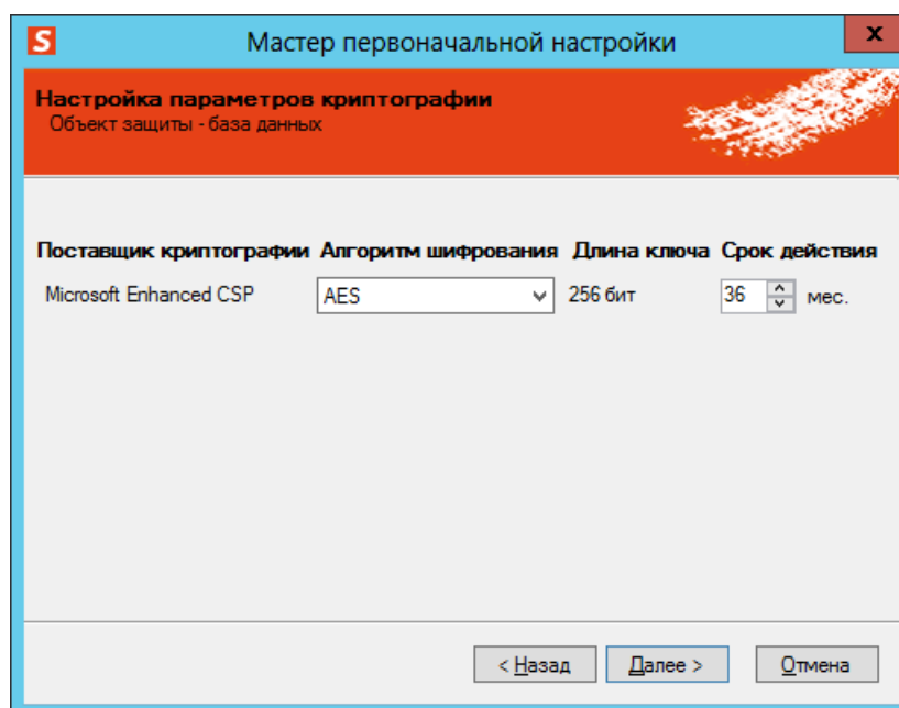
Рис. 89 – Окно настройки параметров криптографии
