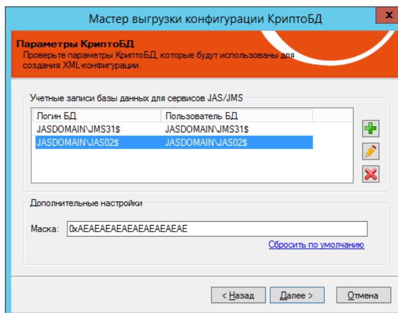
Рис. 245 – Окно задания учетных записей для работы СКЗИ «Крипто БД» с БД IMS
