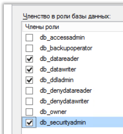
Рис. 255 – Назначение ролей администратору безопасности СКЗИ «Крипто БД» для БД JMS
