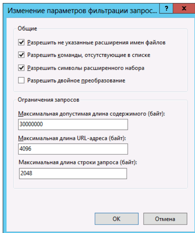
Рис. 8 – Изменение параметров фильтрации запросов
